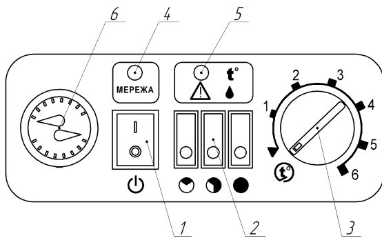
Рисунок 2 Вид панелі керування
