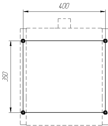
Рисунок 3 Розмітка отворів для кріплення
