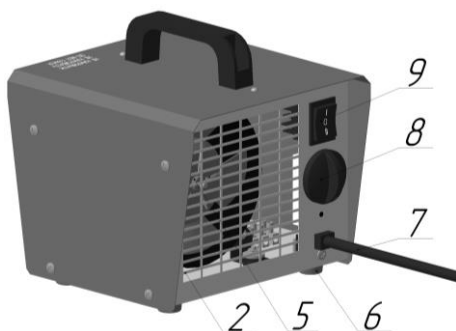
Рисунок 2 Загальний вигляд агрегату
